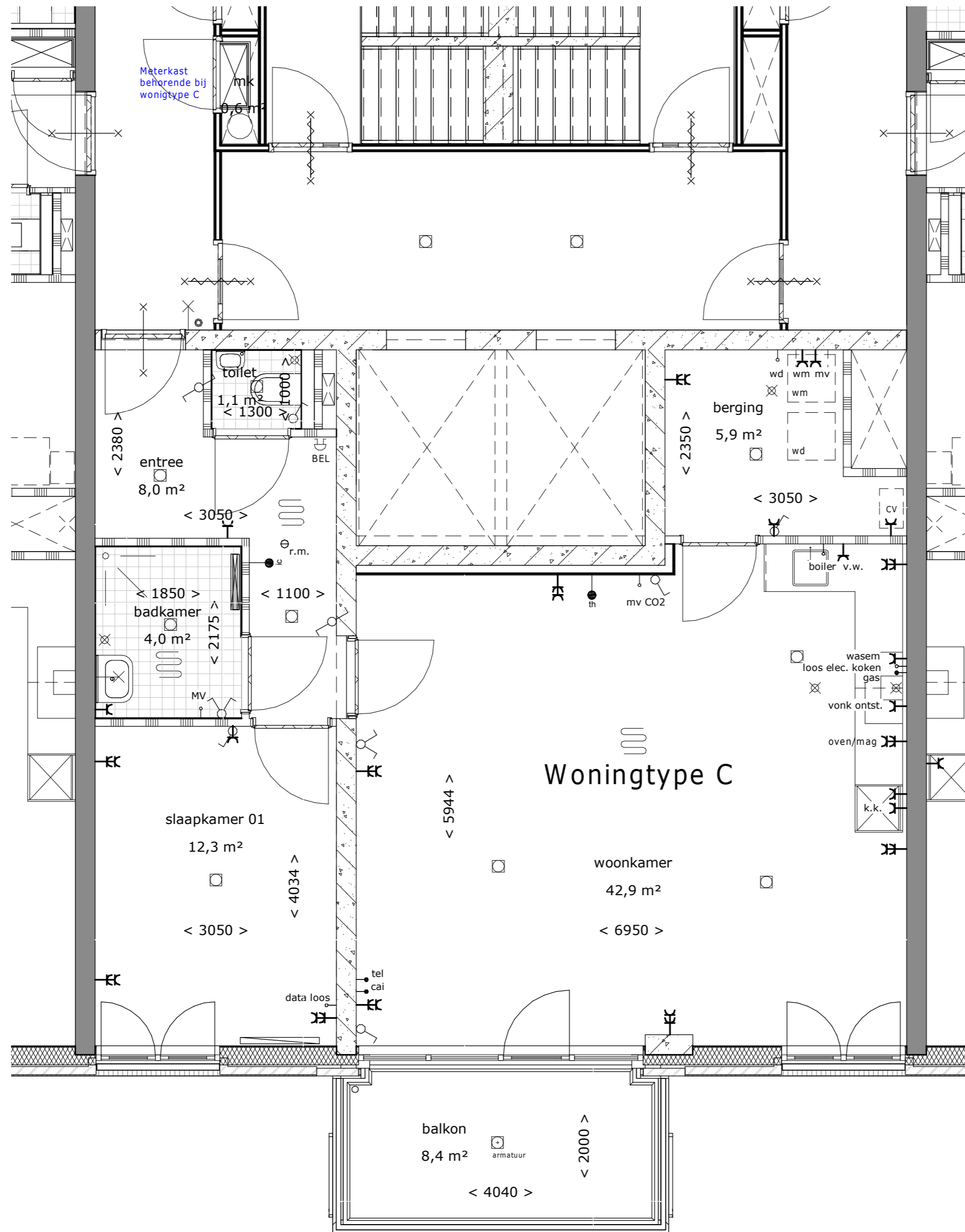
Koopplattegrond -- type C Schaal 1:50
