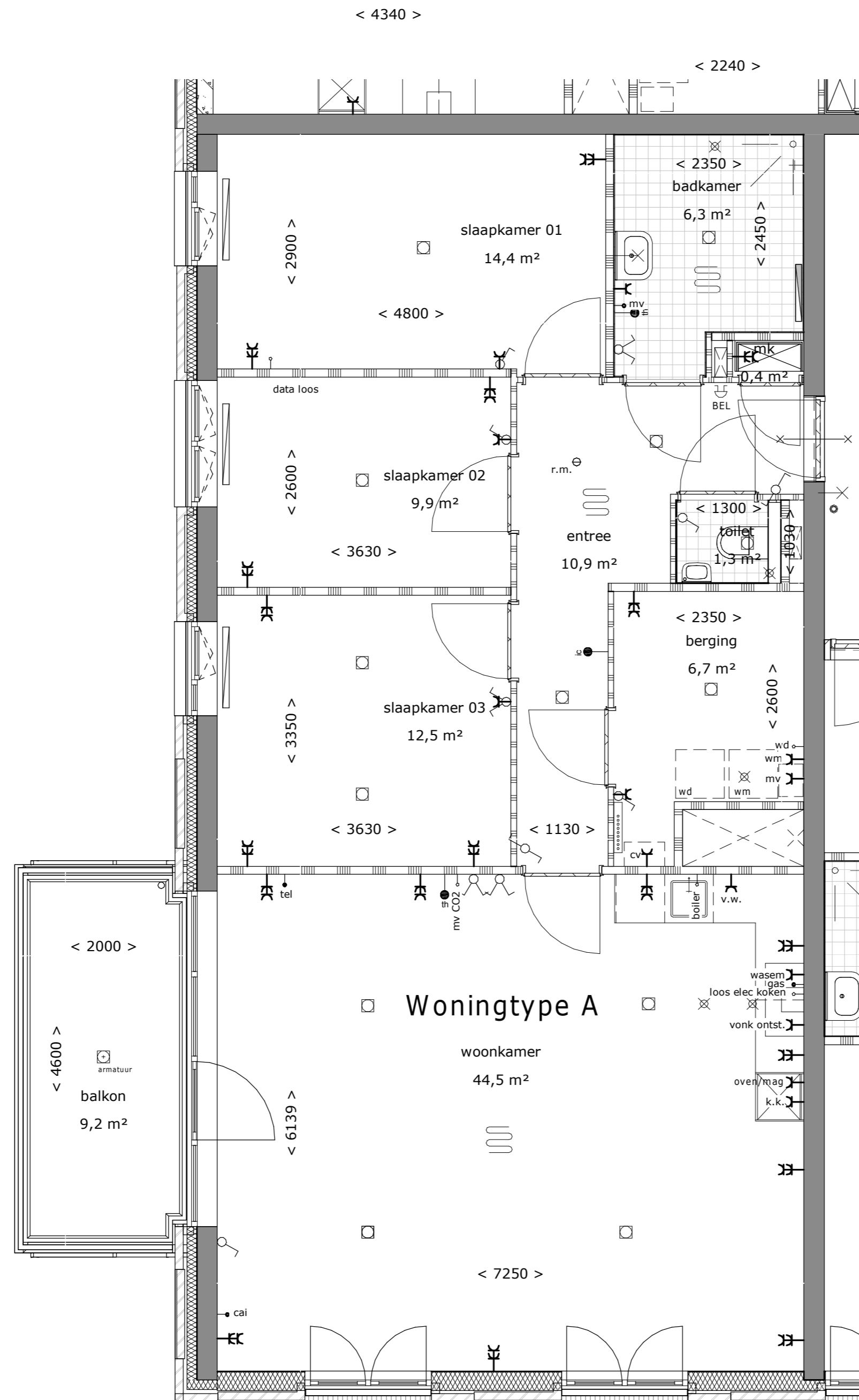
Koopplattegrond -- type A Schaal 1:50
