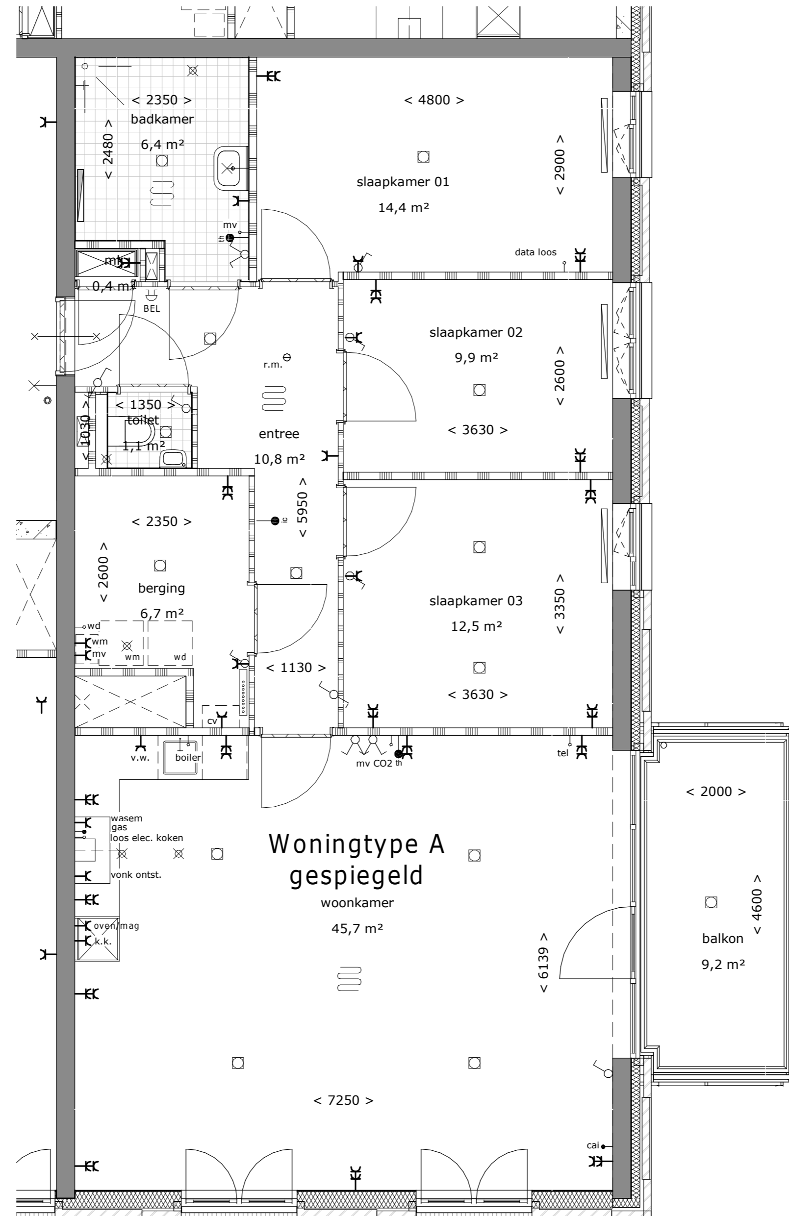
Koopplattegrond -- type A, gespiegeld Schaal 1:50
